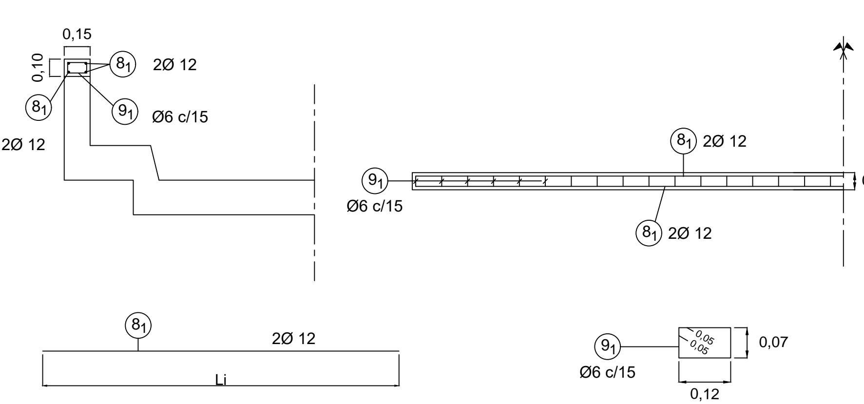
DETALLE ARMADURA BARANDA
