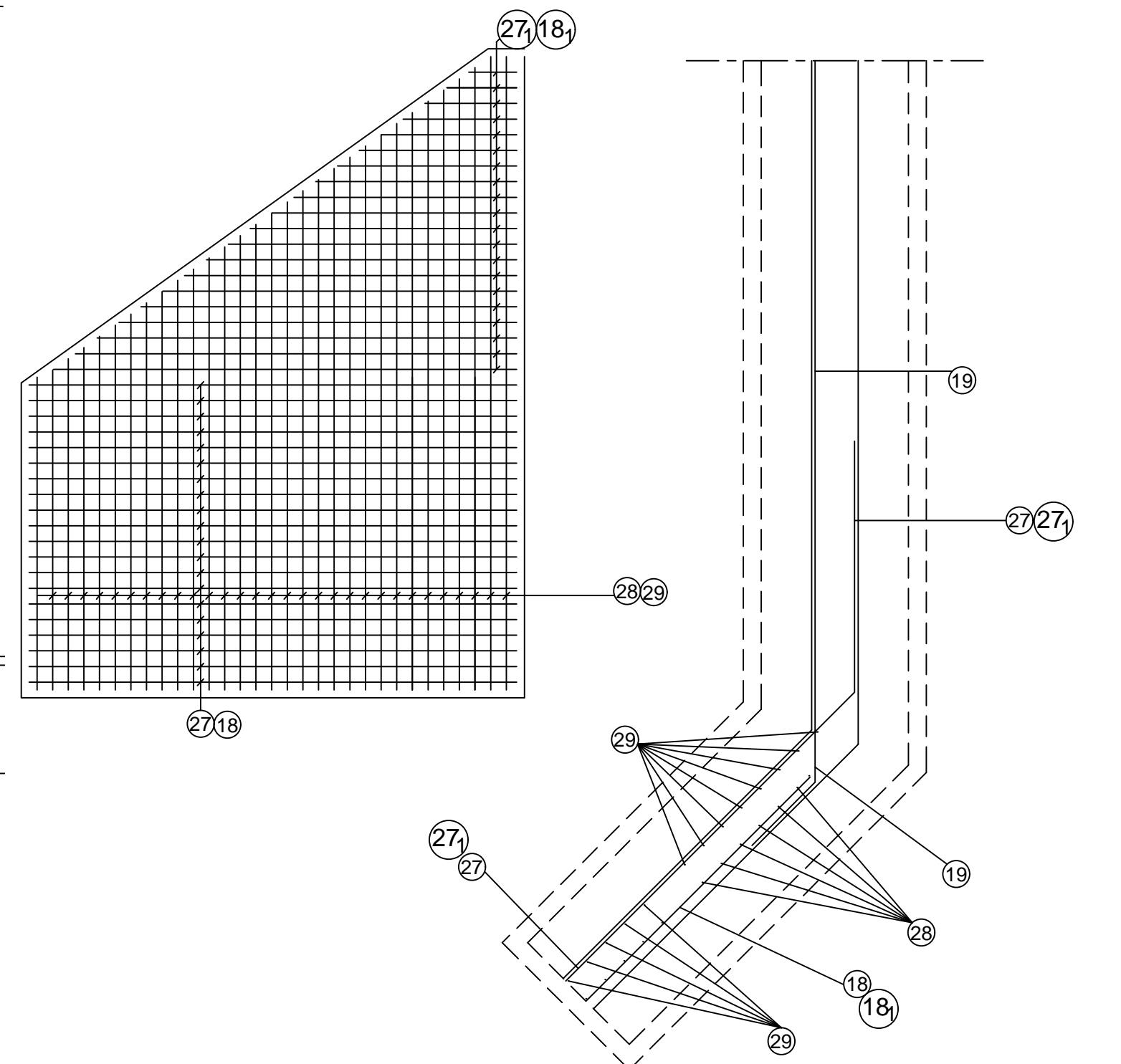
SECCION TRANSVERSAL TABLERO - ARMADURAS
