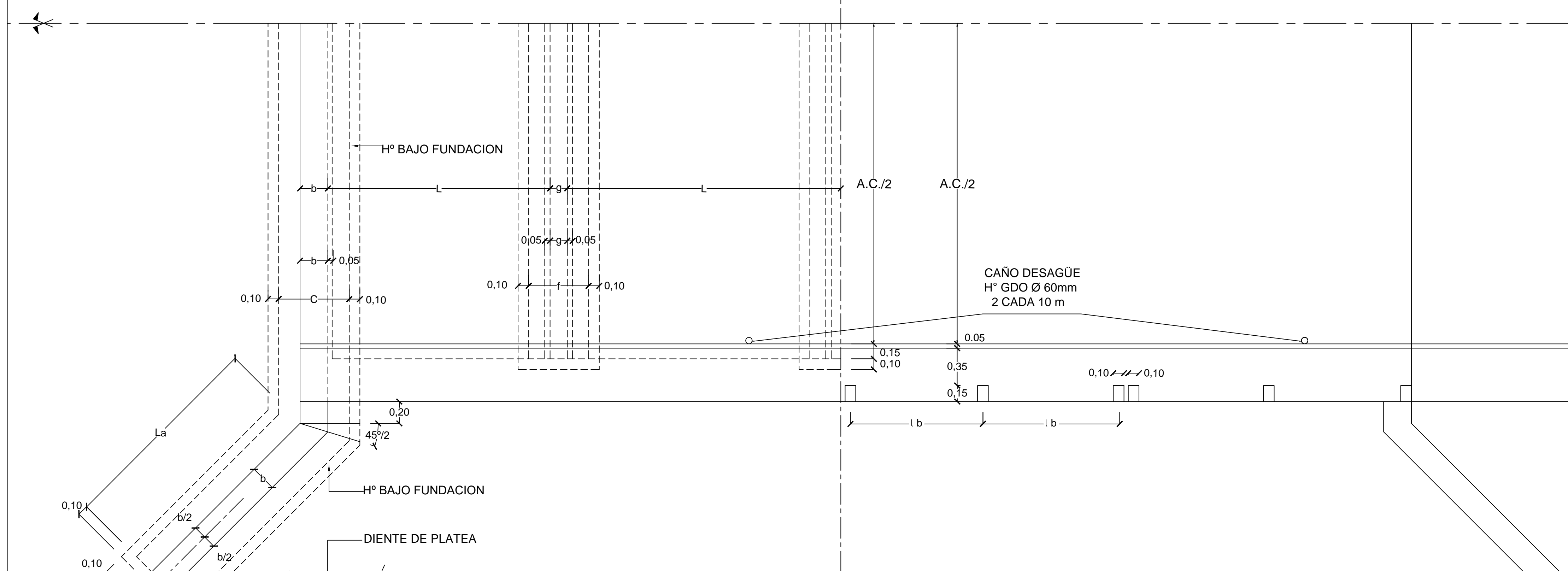
SECCION TRANSVERSAL TABLERO ESCALA 1:25
