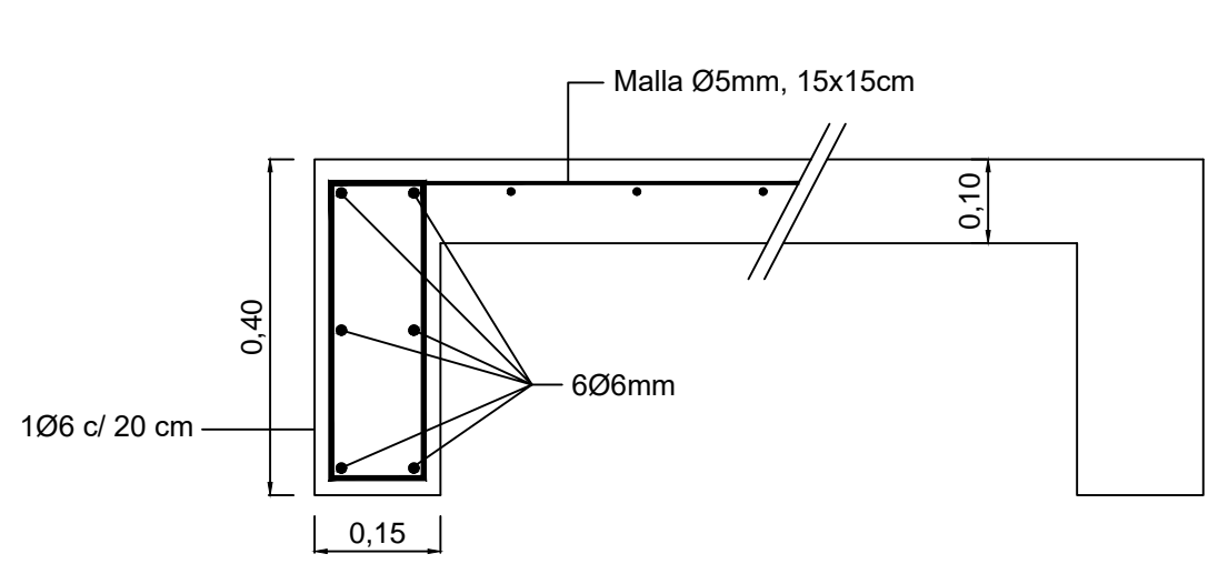
DETALLE PLATEA
