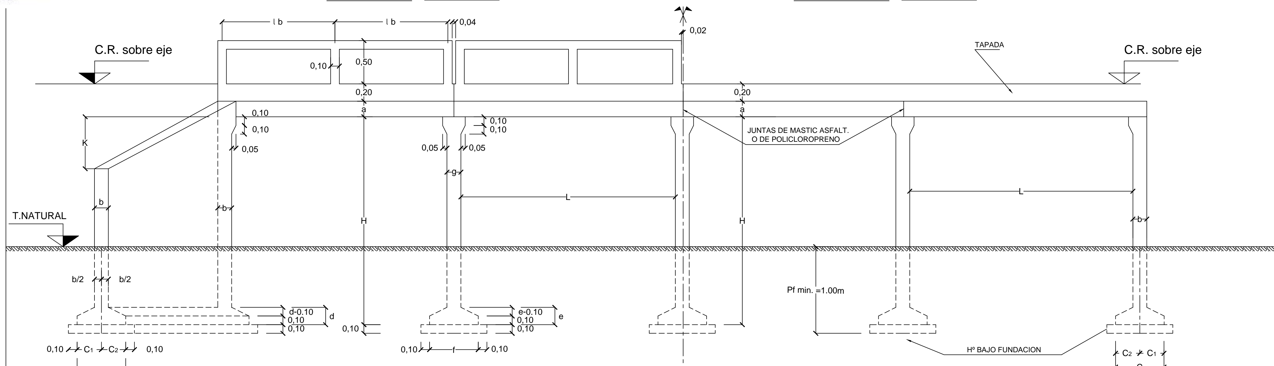
SEMI-CORTE ESCALA 1:25
