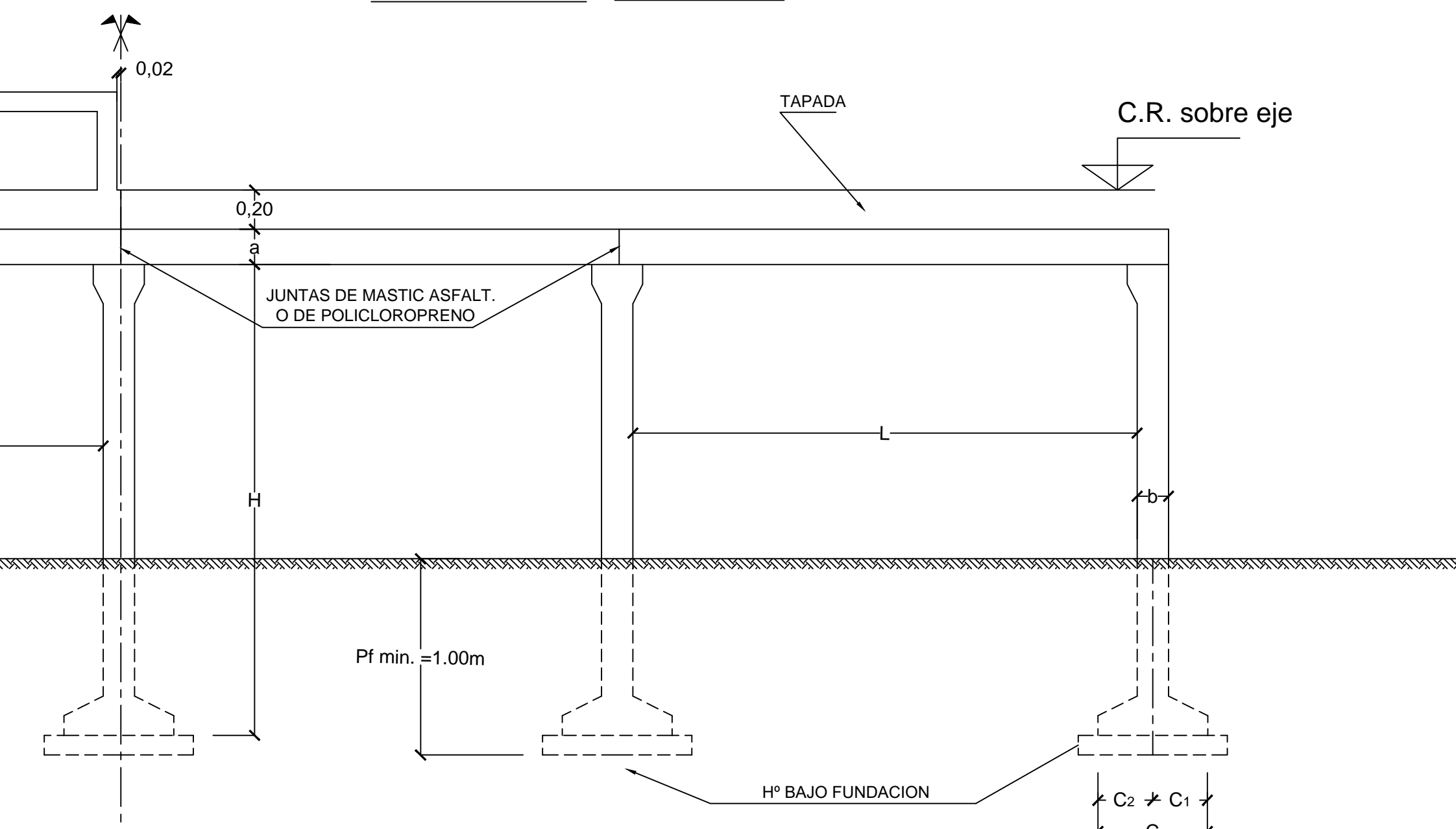
SEMI-CORTE ESCALA 1:25
