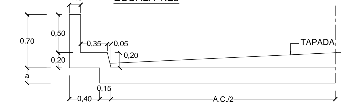
SECCION TRANSVERSAL TABLERO ESCALA 1:25
