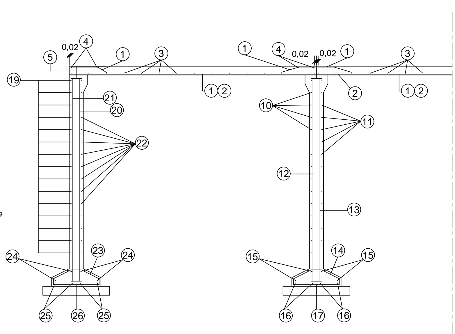
DETALLE ARMADURAS MURO DE ALA
